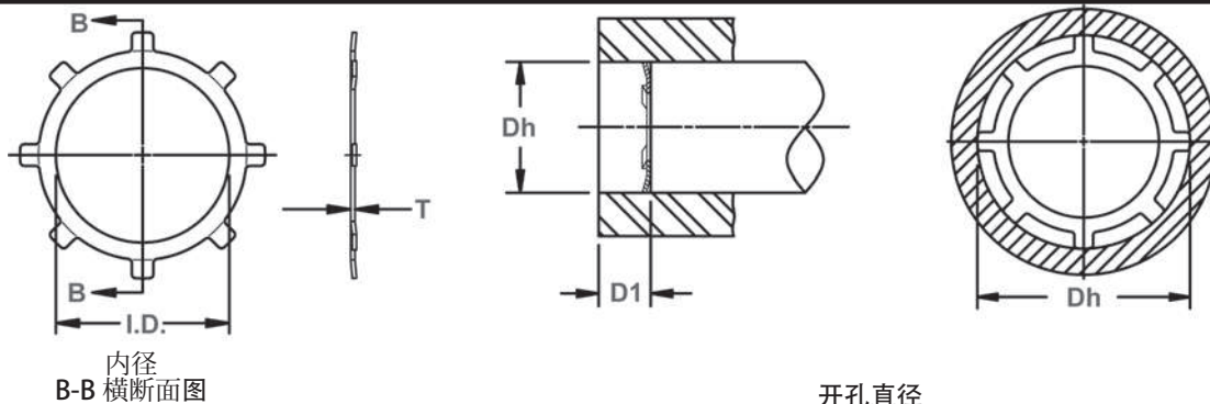
开孔直径
