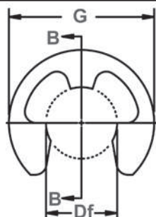
自由直径&扣环尺寸 B-B 横断面图
